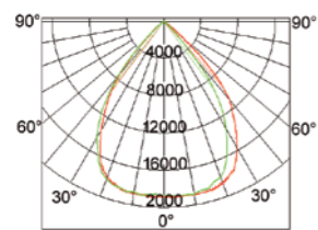
配光図
